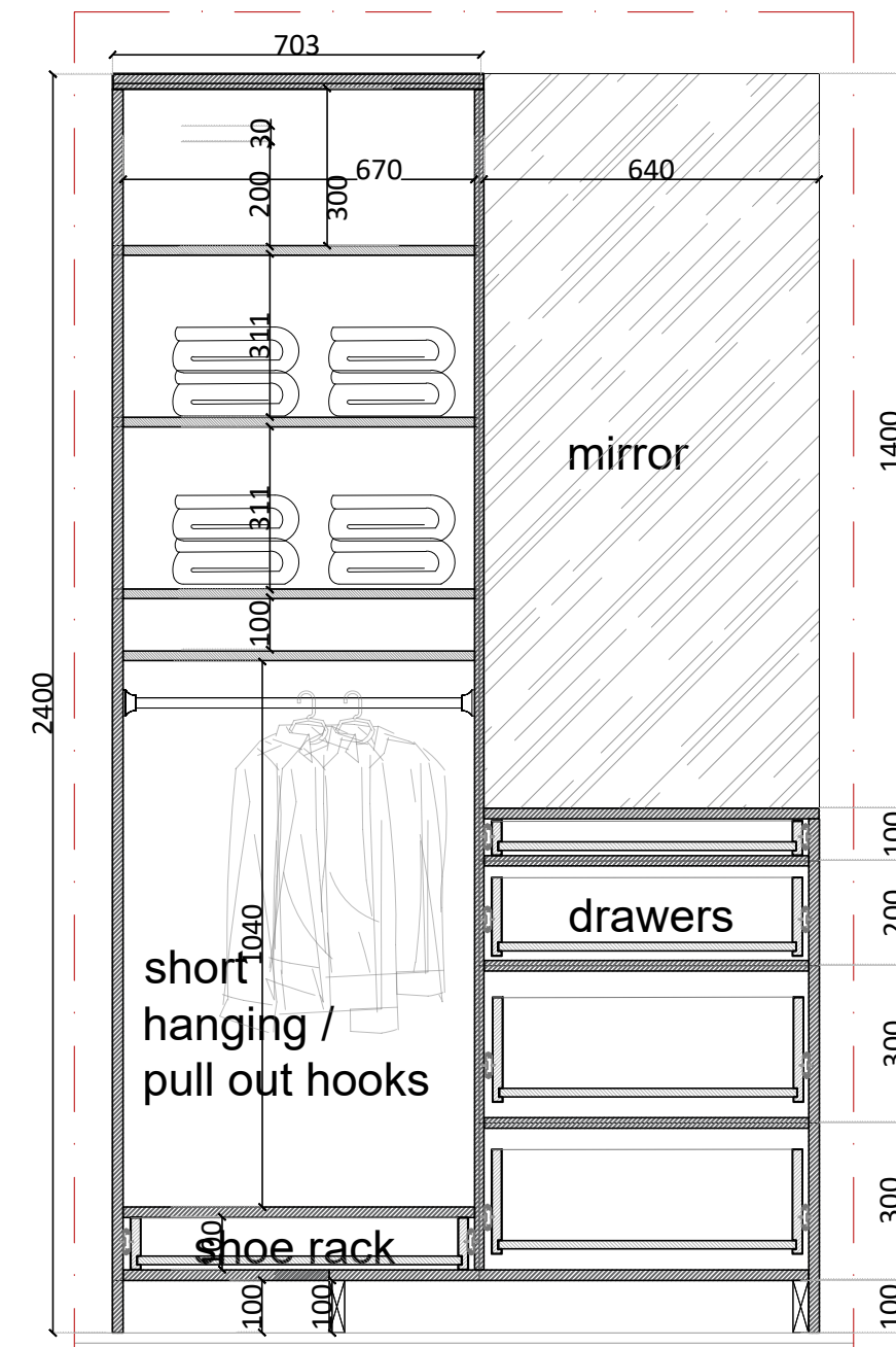
03 SECTION AA JW-MR-25
