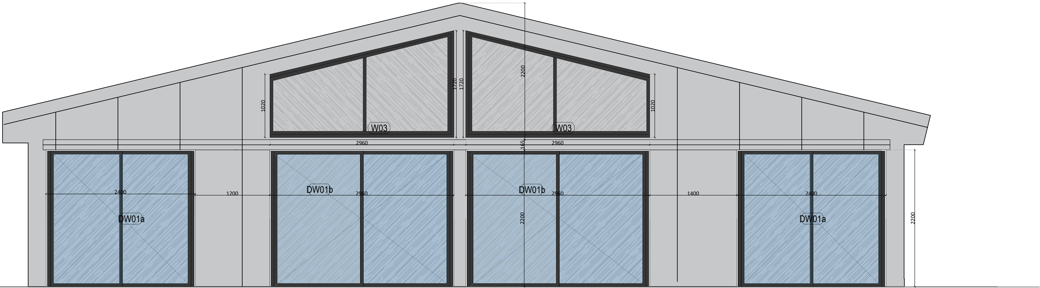
02 | ELEVATION D
