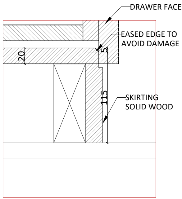
06 DT 01
