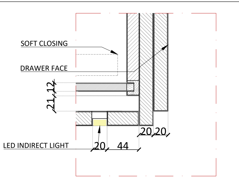
08 | DETAIL 01 JW-MB-14
