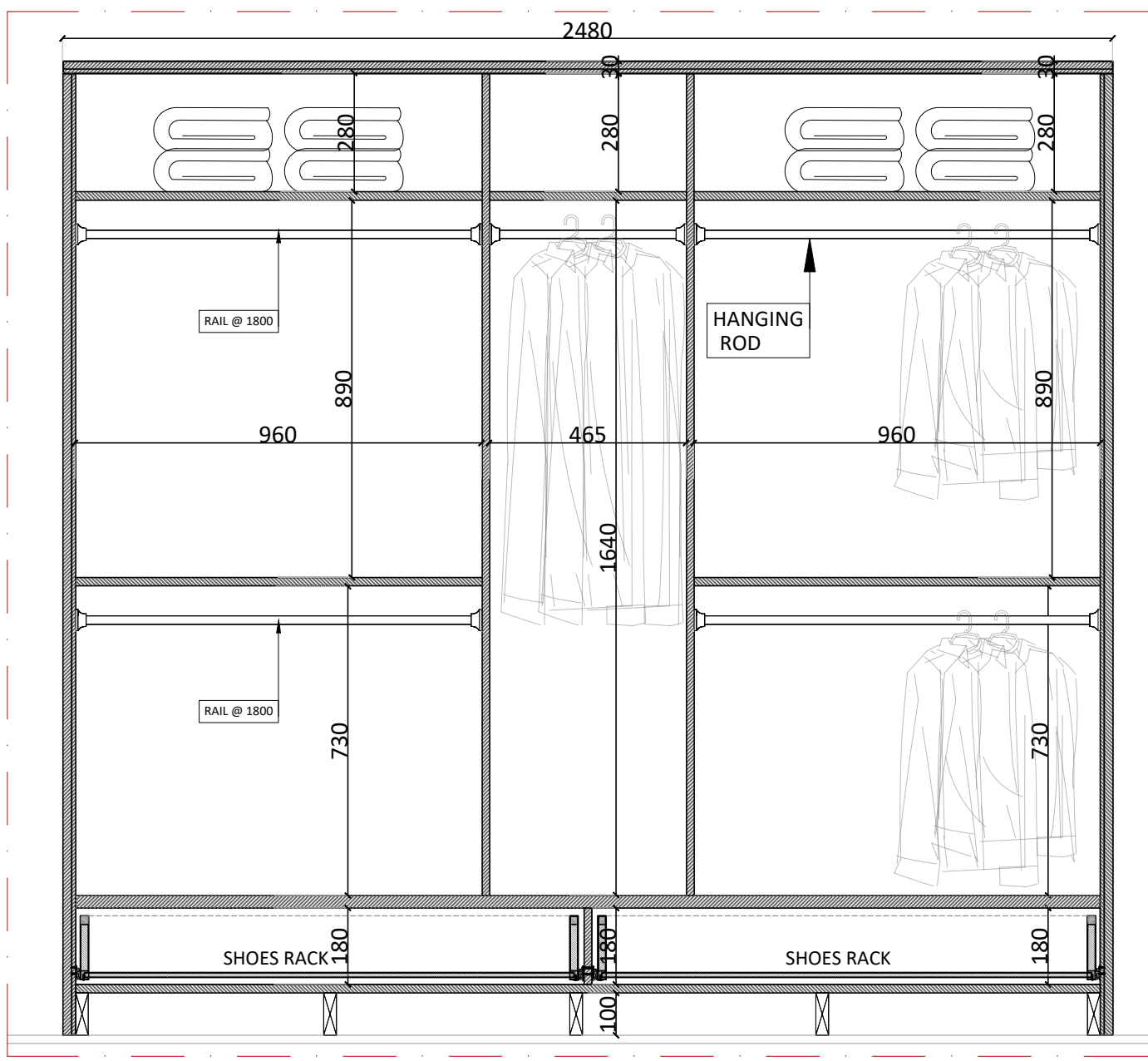
03 SECTION A JW-MB-13
