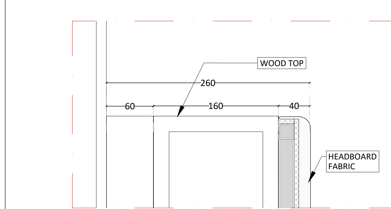
05 D1
