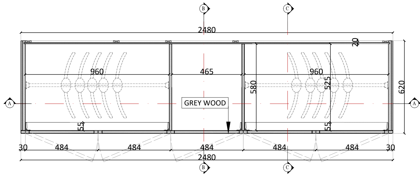
01 WARDROBE JW-MB-13 PLAN
