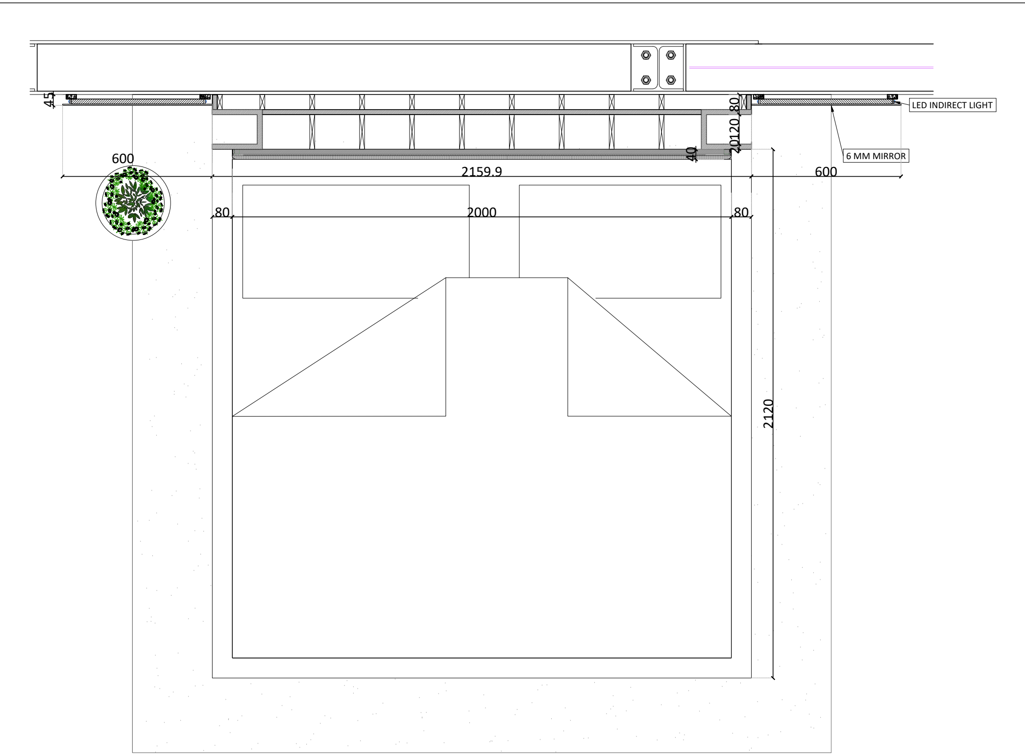
05 D1
